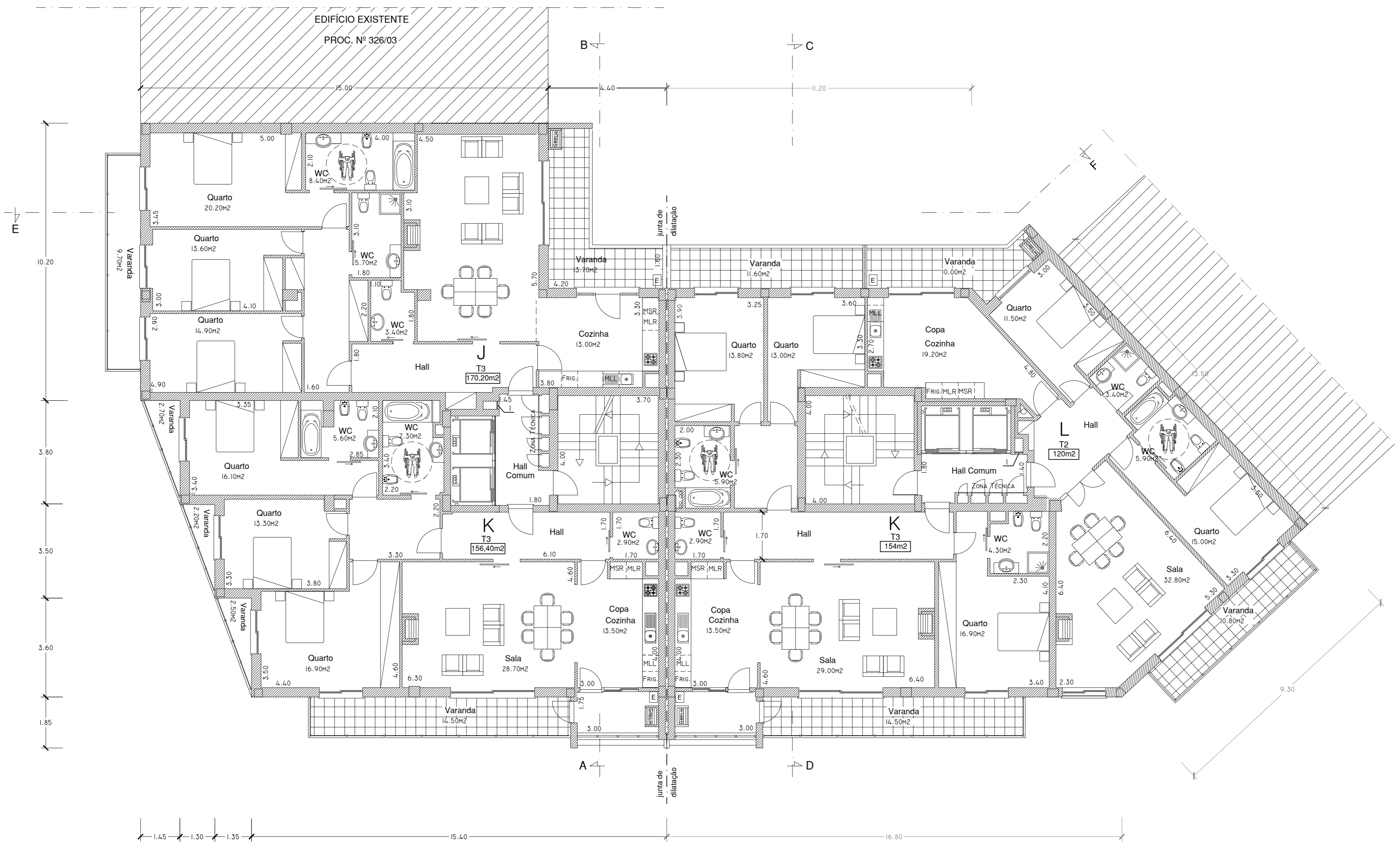
PLANTA DO 5º ANDAR
