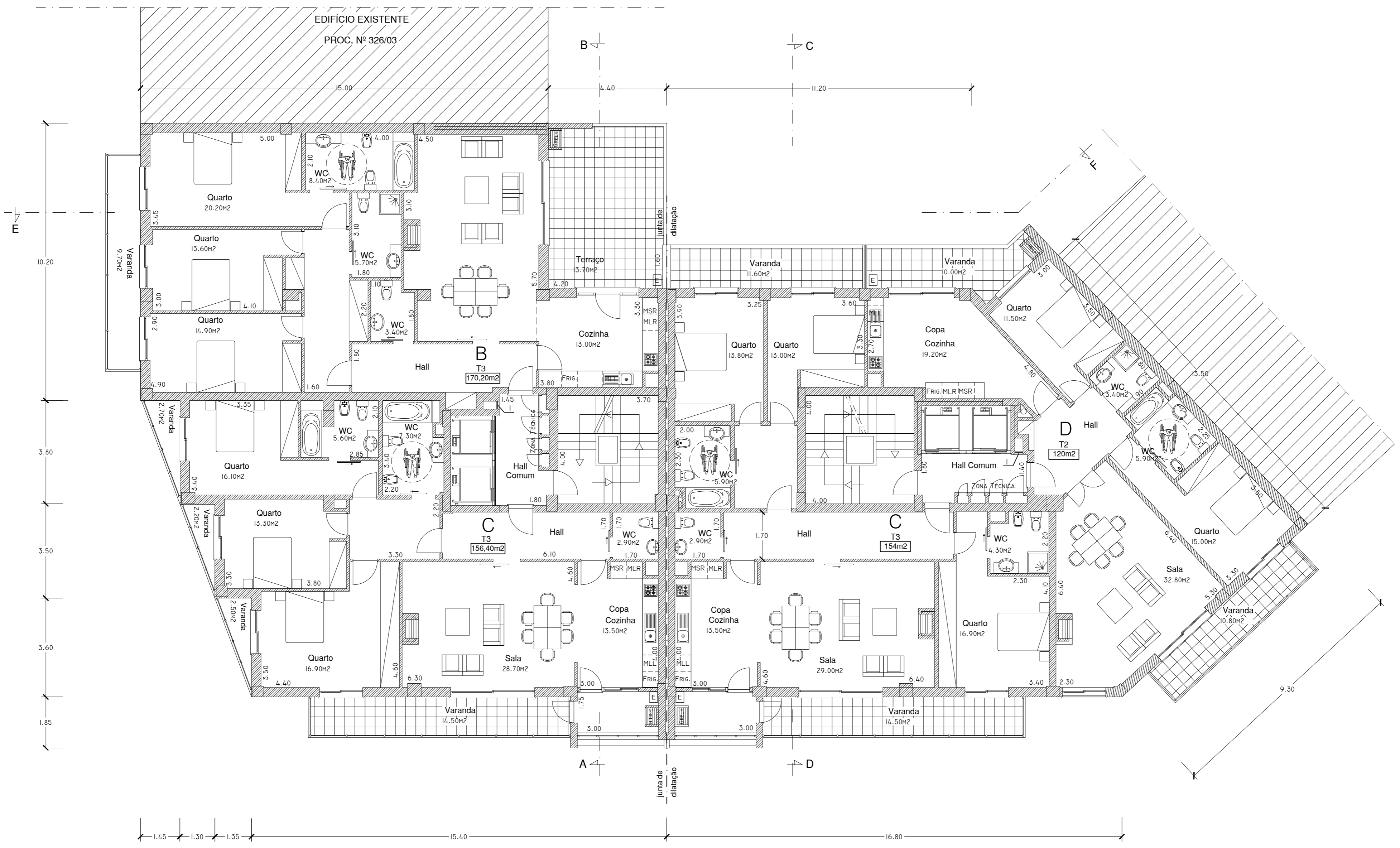
PLANTA DO 1º ANDAR
